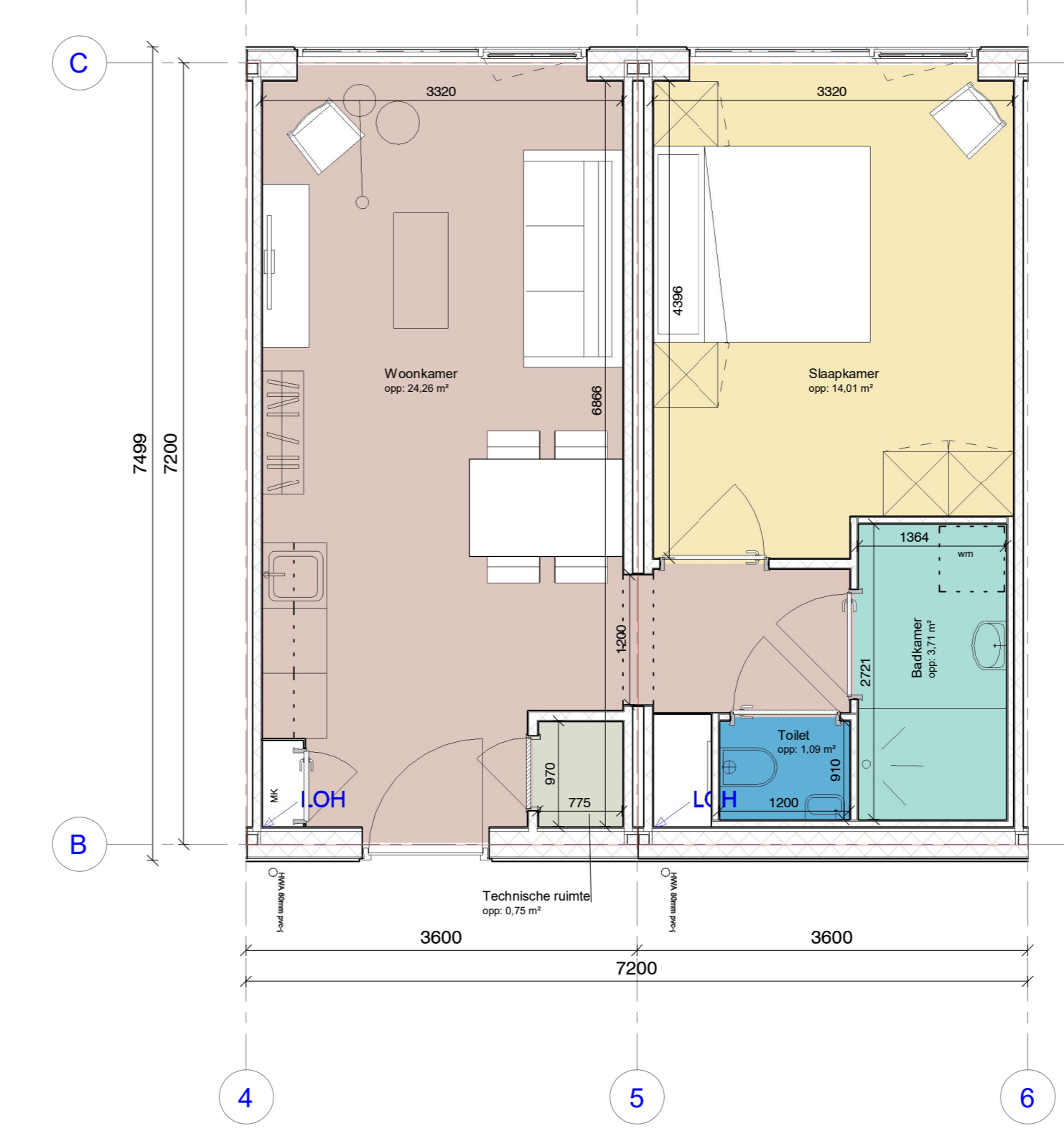
Single+ / twee kamer woning schaal 1 : 50
