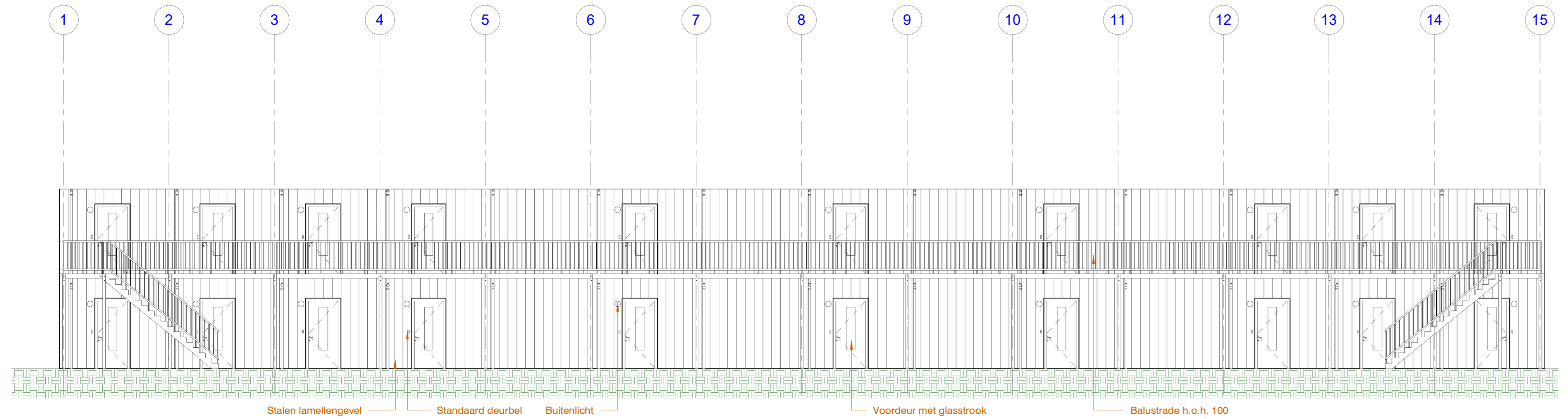
Voorgevel schaal 1 : 100
