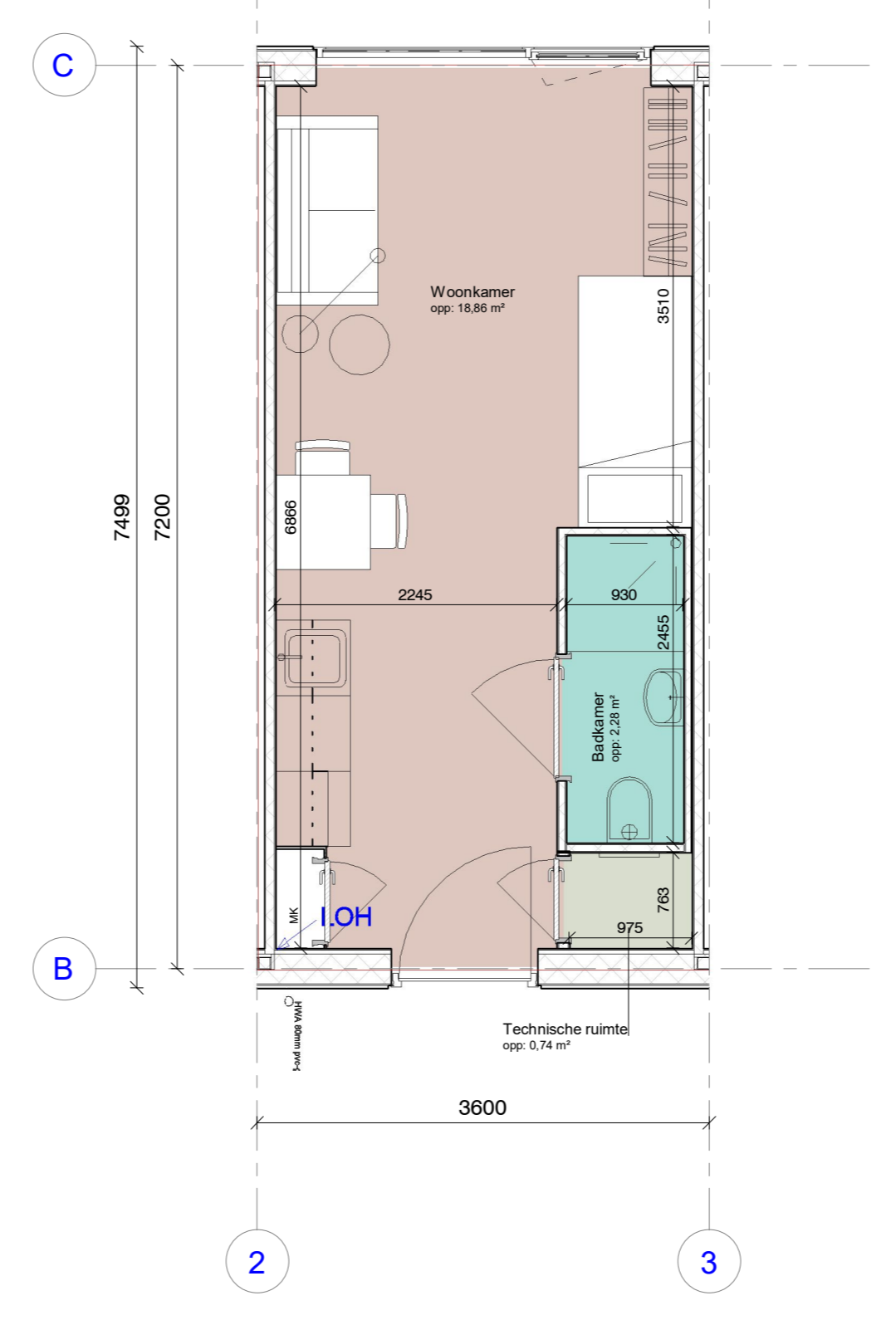
Studio+ / één kamer woning schaal 1 : 50
