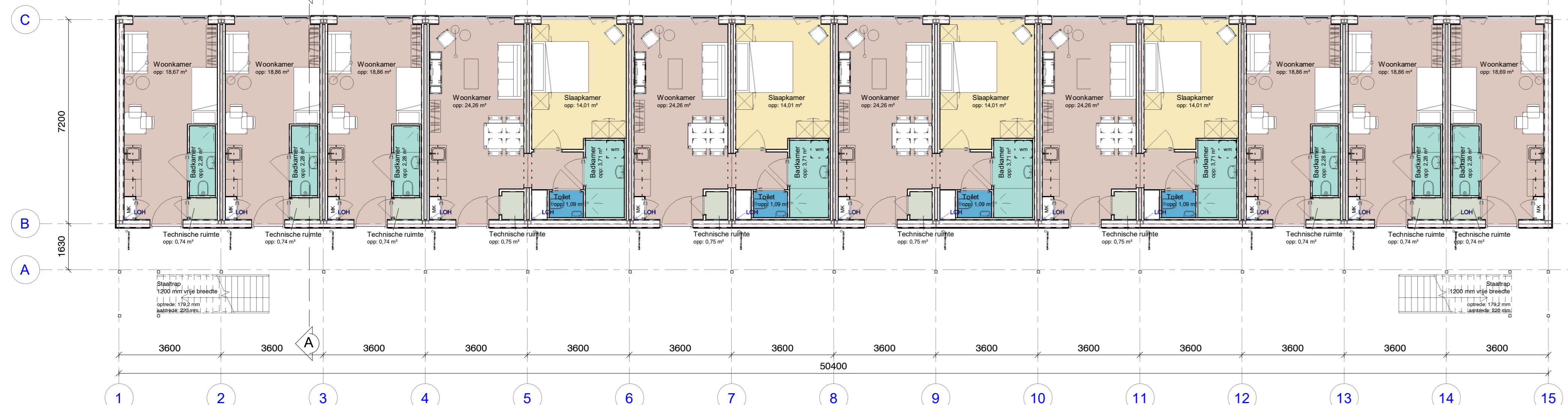
Begane grond schaal 1 : 100
