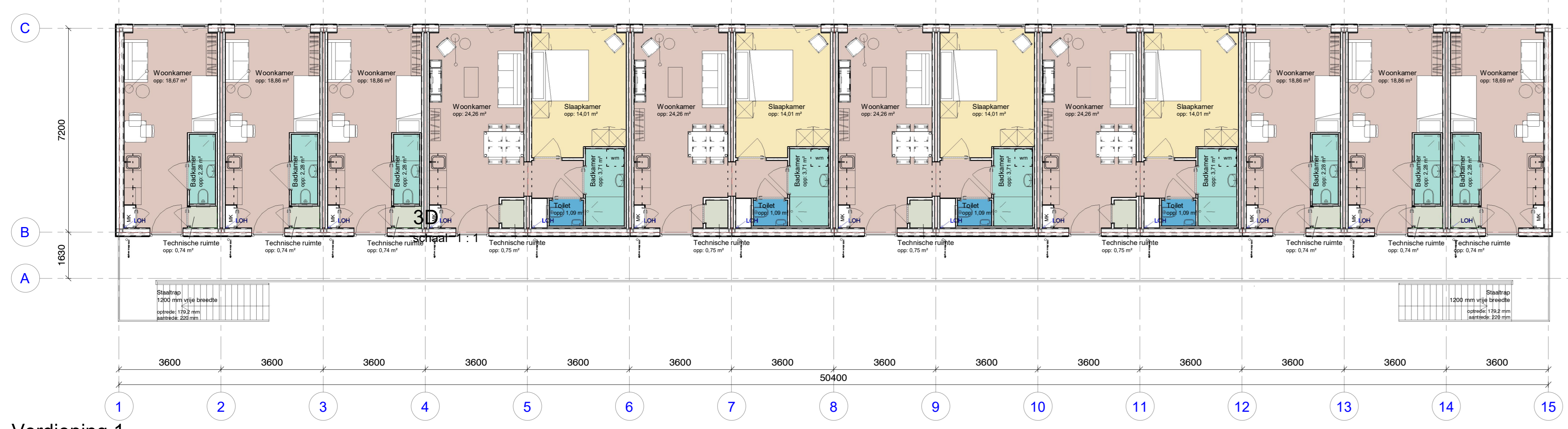
Verdieping 1 schaal 1 : 100
