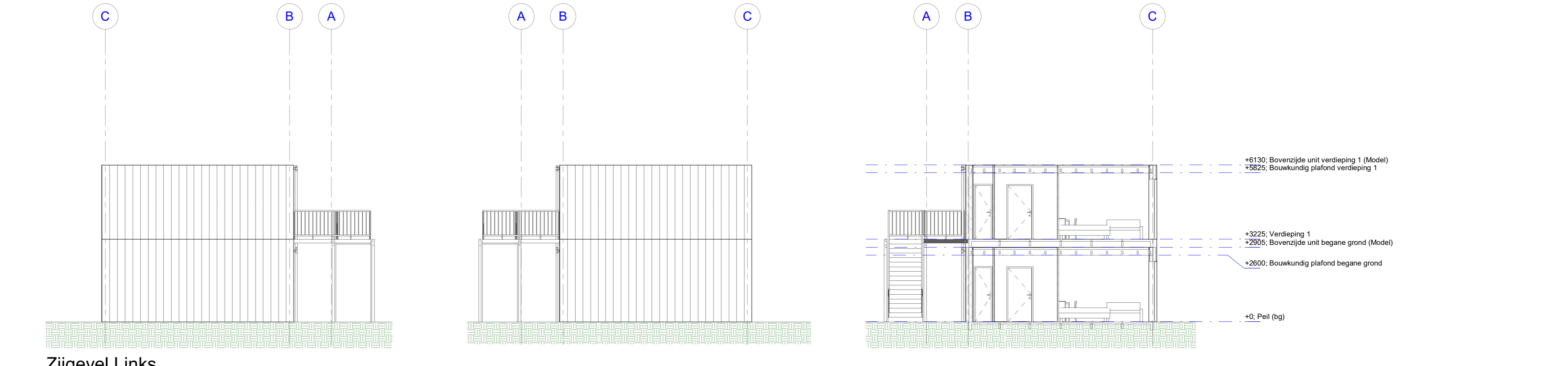
Zijgevel Links schaal 1 : 100 Zijgevel Rechts schaal 1 : 100 Doorsnede A-A (VO-plt) schaal 1 : 100
