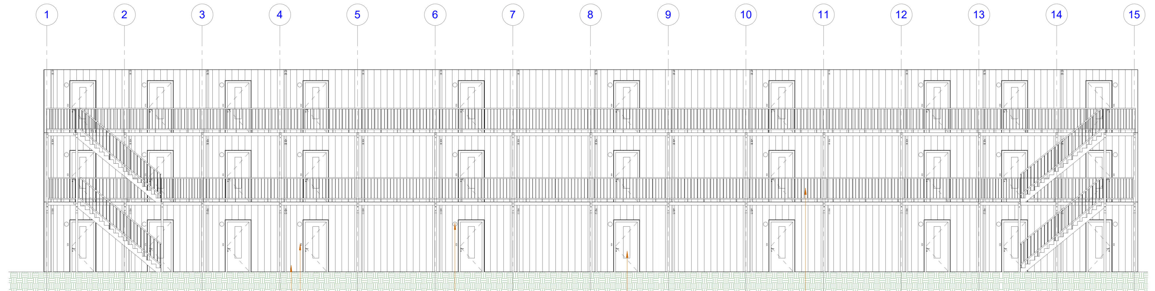
Voorgevel schaal 1 : 100
